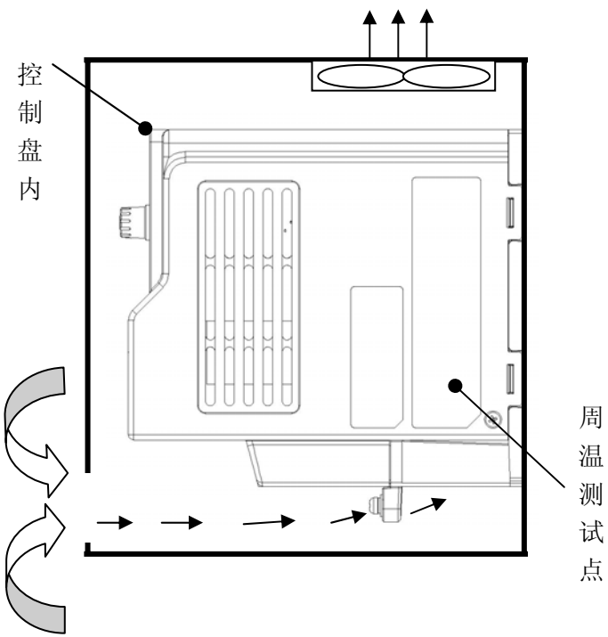
侧面
